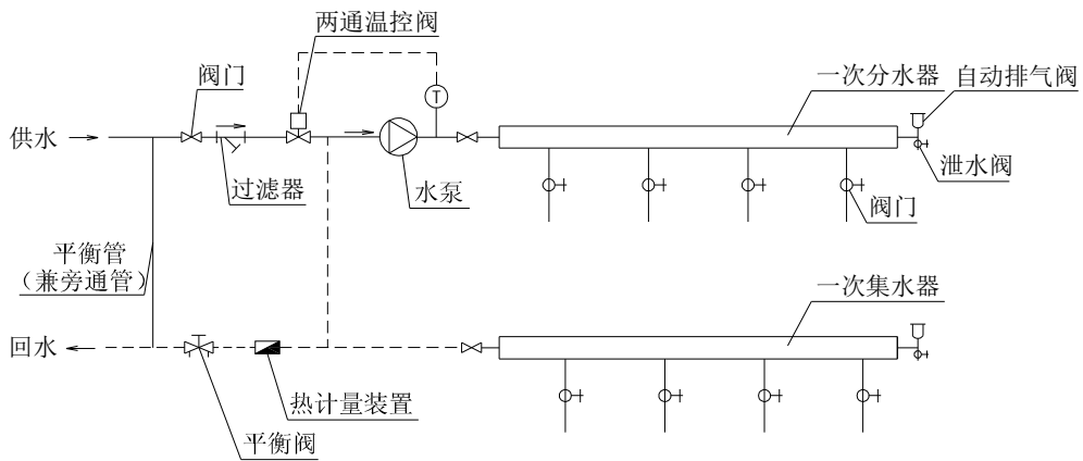
图 E. 0. 3-2 采用两通阀的混水系统
