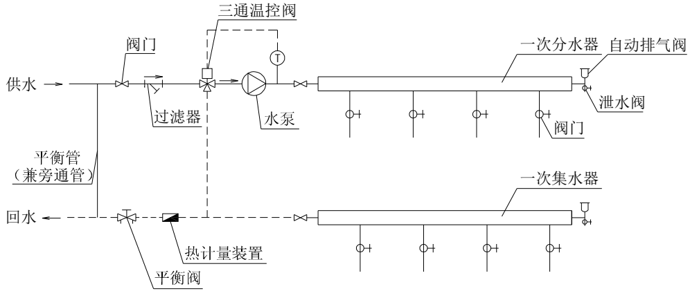
图 E. 0. 3-1 采用三通阀的混水系统
