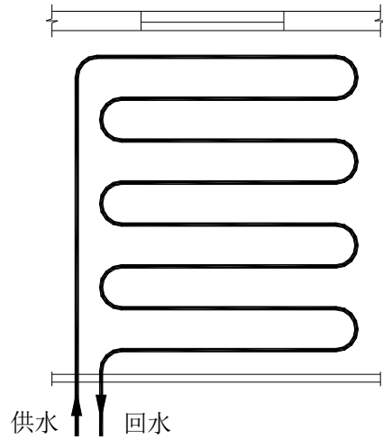
图 F.0.1-2 平行型布置
