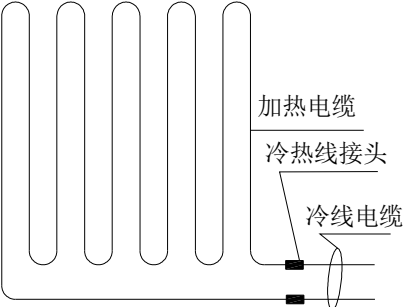
图 F.0.2-1 单导加热电缆单路平行布置
