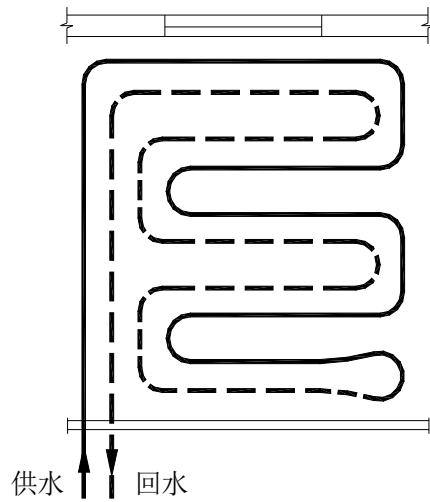
图 F.0.1-3 双平行布置
