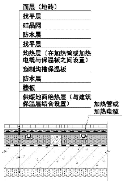
图A.2.4 预制沟槽保温板地面供暖构造(四) (潮湿房间, 与不供暖房间相邻及与室外空气接触的地面)
