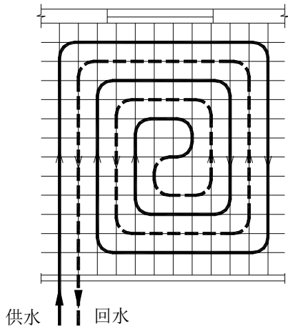
图 F.0.1-1 回折型布置
