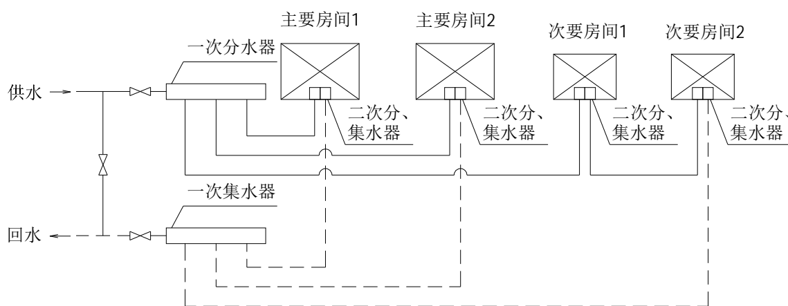
图 D.0.3 供暖板地面供暖系统示意
