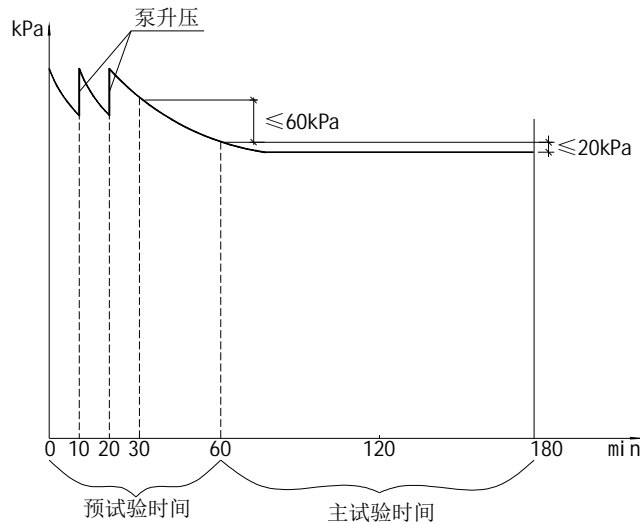
图 7 水压试验时间分配和压力示意
