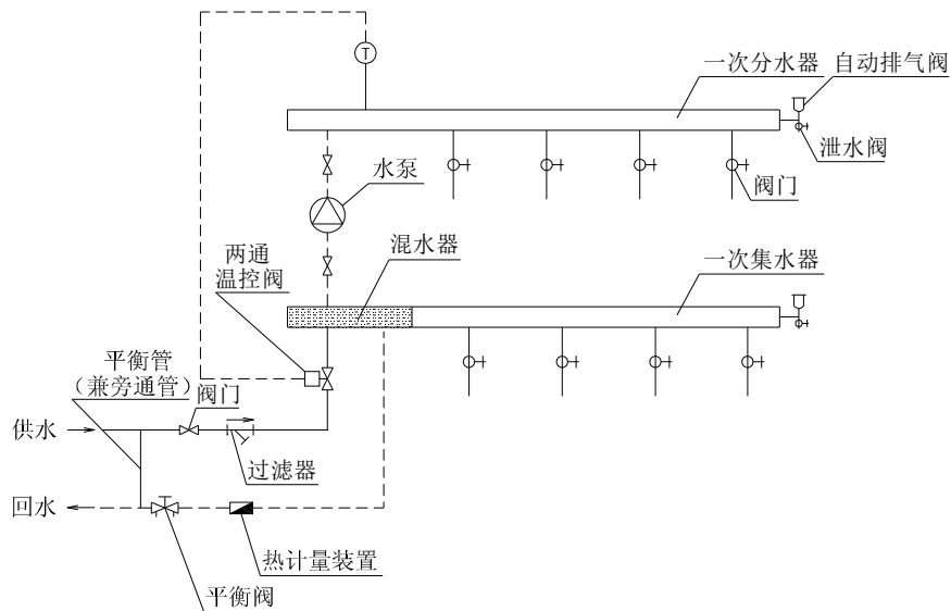
图 E. 0. 3-3 设置混水器的系统
