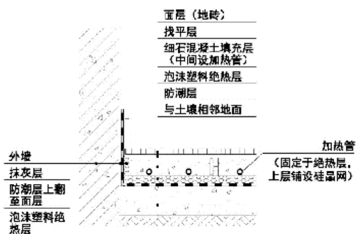
图A.1.2 混凝土填充式地面供暖构造（二）
