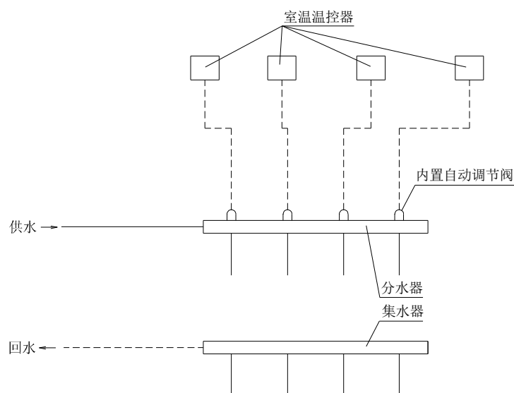
图 I.0.2 分环路（分室）控温示意图
