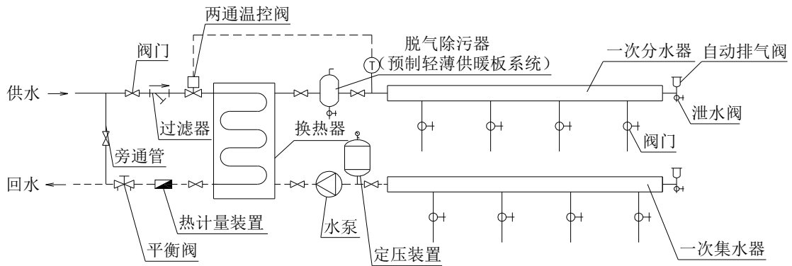
图 E.0.2 间接供暖系统示意图
