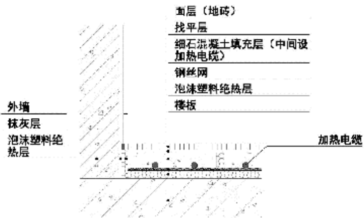
图A. 1. 4 混凝土填充式地面供暖构造 (四) (非潮湿房间, 设加热电缆, 与供暖或不供暖房间相邻及与室外空气接触的地面)
