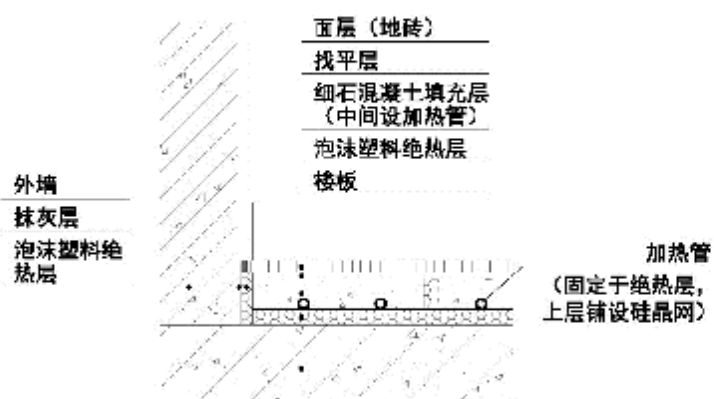
图A.1.1 混凝土填充式地面供暖构造（一）
