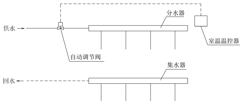
图 I.0.1 总体（分户）控温示意图
