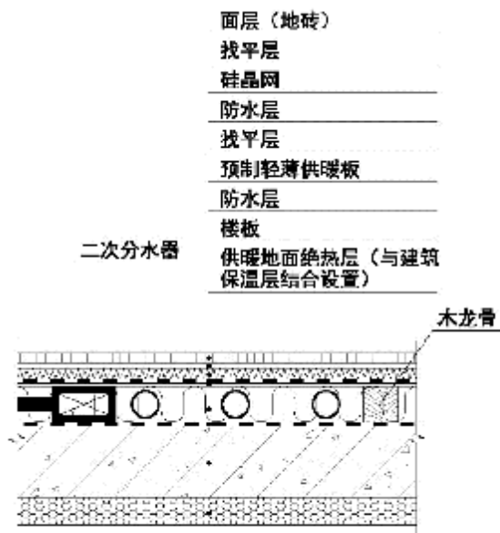
图A. 3.4 预制轻薄型供暖板地面供暖构造（四） （潮湿房间，与不供暖房间相邻及与室外空气接触的地面）
