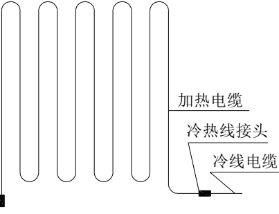
图 F.0.2-2 双导加热电缆平行布置
