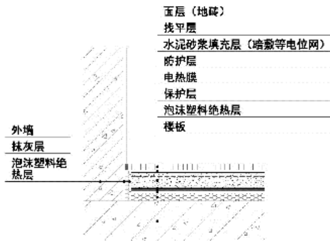
图A. 1.7 混凝土填充式地面供暖构造（七）
