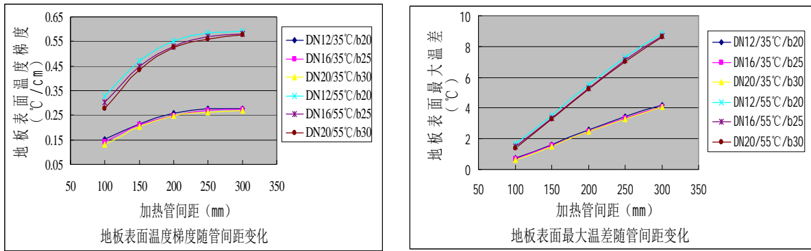
图5 不同管间距地板表面的温度梯度和最大温差
