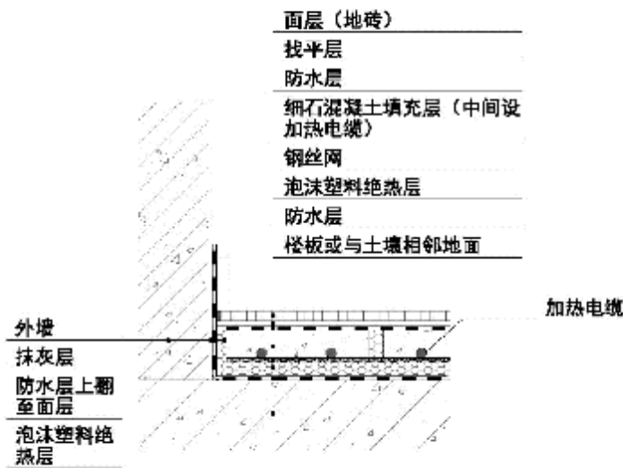
图A. 1. 6 混凝土填充式地面供暖构造（六）
