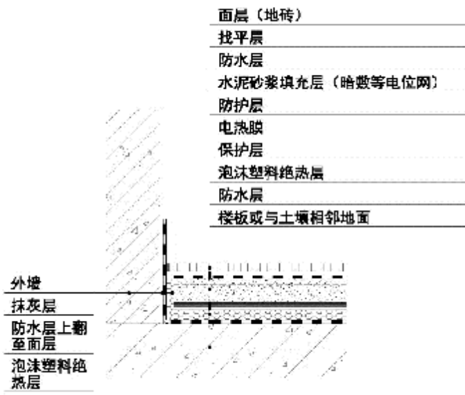
图A. 1. 9 混凝土填充式地面供暖构造 (九)
