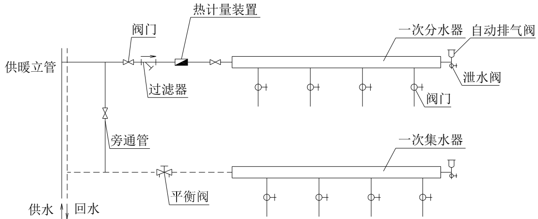
图 E.0.1 直接供暖系统示意图
