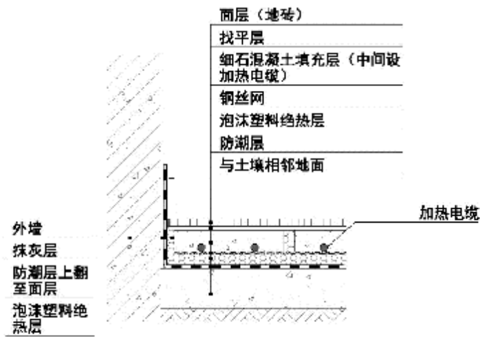
图A. 1. 5 混凝土填充式地面供暖构造（五）
