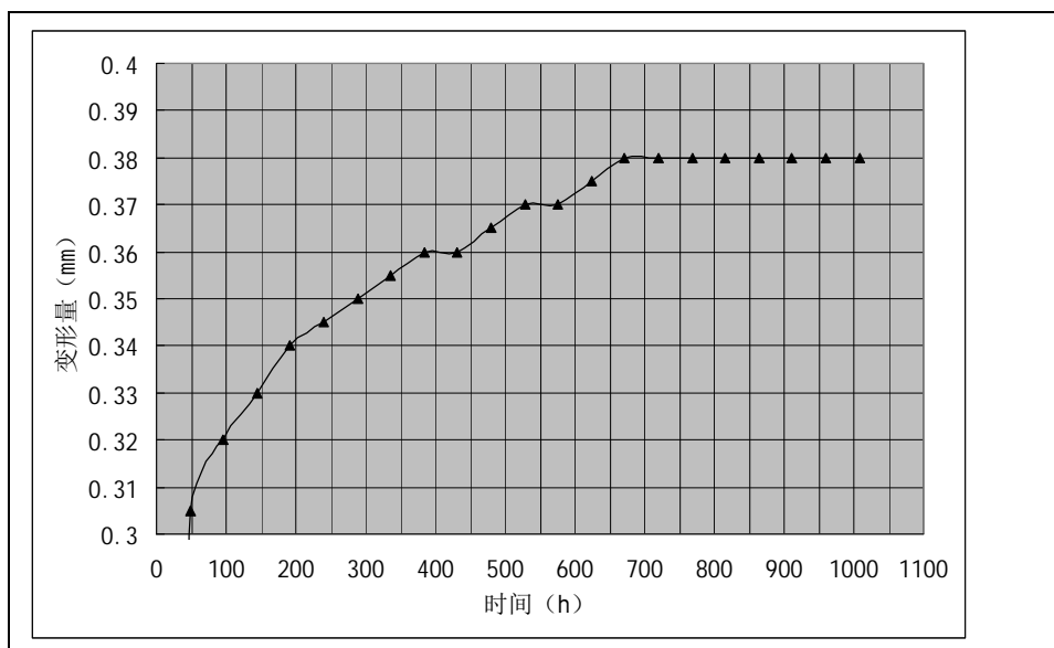
图 4 预制轻薄供暖板长期局部荷载试验结果
