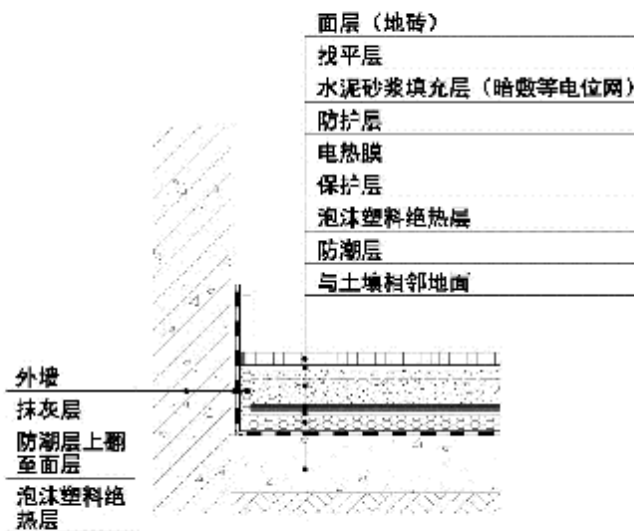
图A. 1.8 混凝土填充式地面供暖构造（八）
