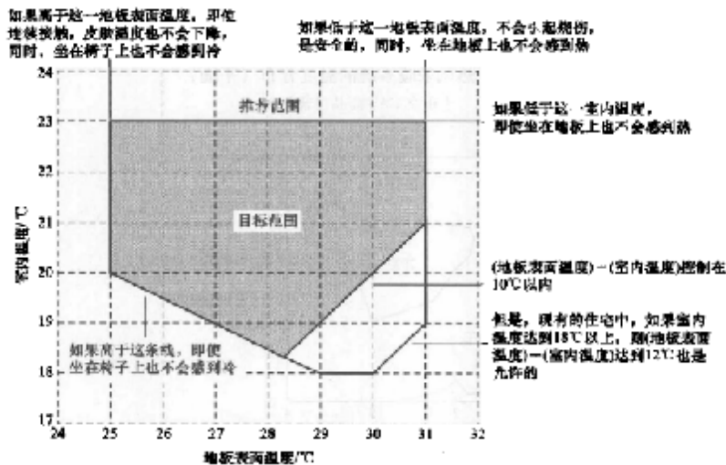
图 1 《床暖房設計・施工マニュアル》推荐的地面供暖舒适度范围
