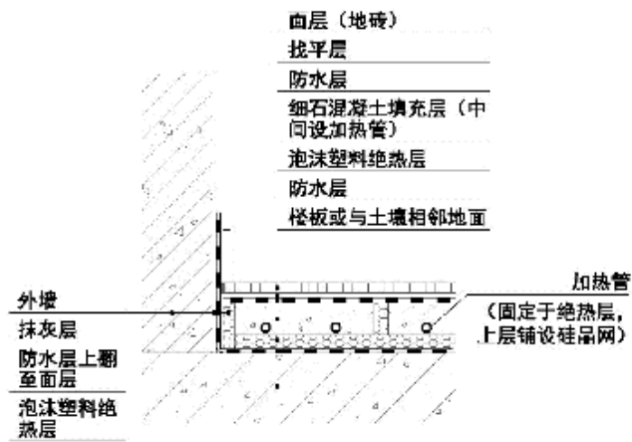
图A. 1. 3 混凝土填充式地面供暖构造 (三) (潮湿房间, 设加热管的地面)
