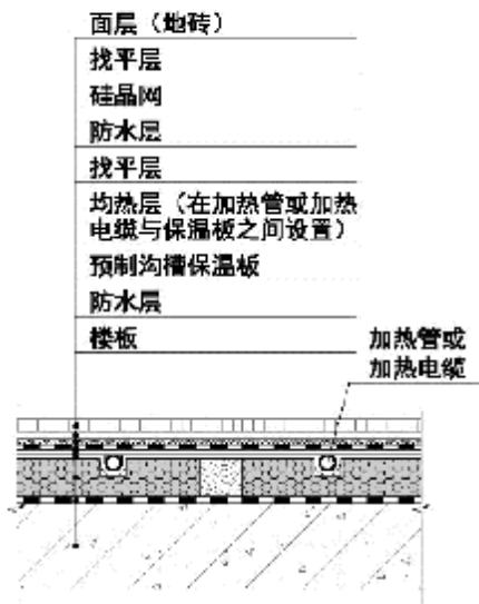
图A.2.3 预制沟槽保温板地面供暖构造(三) (潮湿房间, 与供暖房间相邻的地面)
