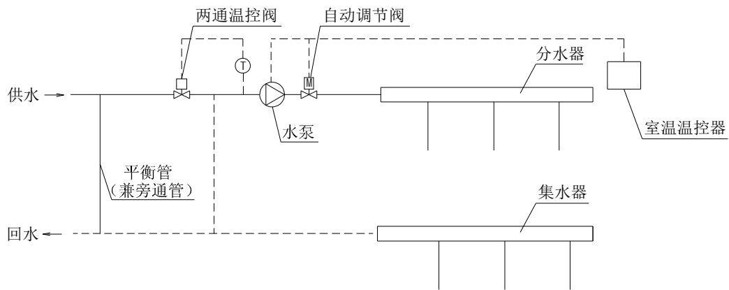
图 I.0.3 混水系统分户控温示意图
