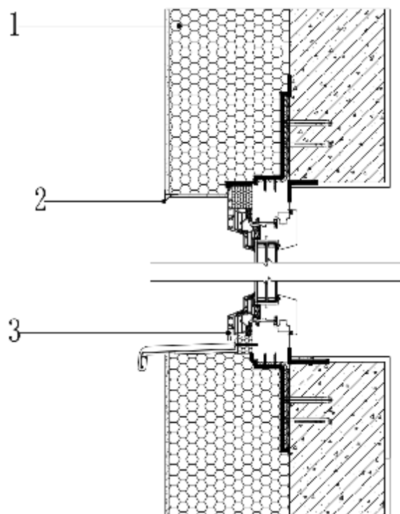
图 B.0.10 窗洞口保温做法剖面图
