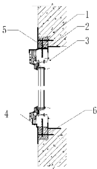
图 B.0.17 外窗带隔热附框的洞内安装方式
