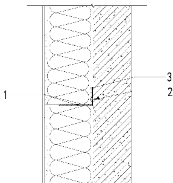
图 B.0.6 层间或起步托架安装
