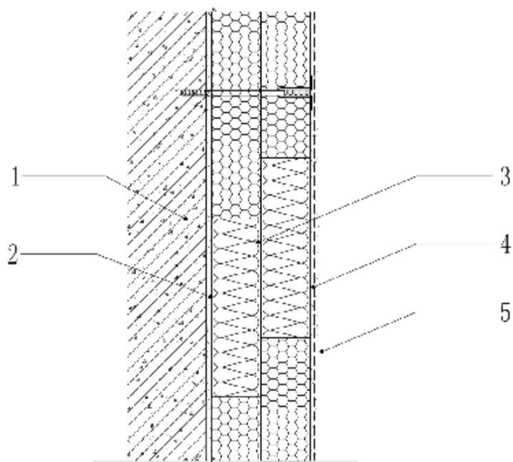
图 B.0.8 防火隔离带分层铺贴
