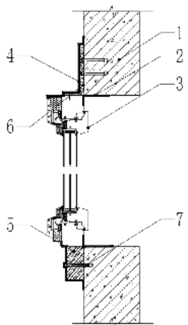
图 B.0.16 外窗外挂式安装-底部采用支撑块
