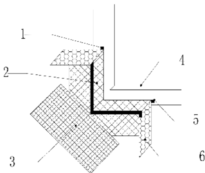
图 B.0.9 窗框外侧保温做法
