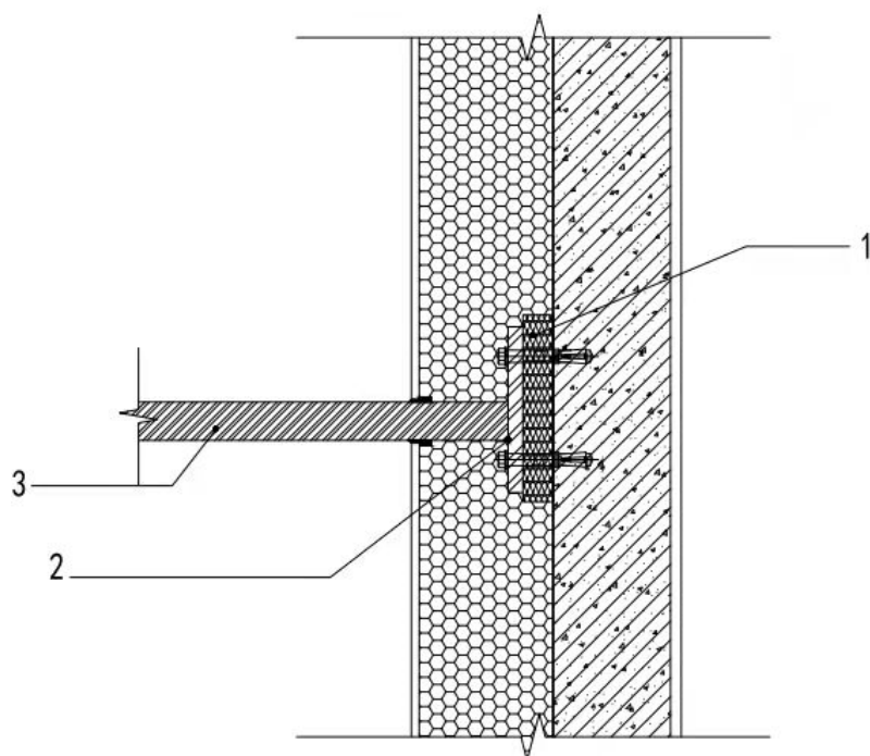
B.0.5 空调支架做法示意图
