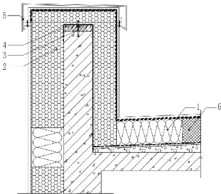
图 B.0.14 女儿墙保温及压顶板做法
