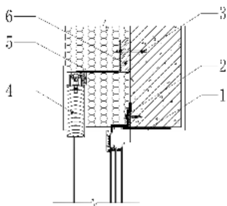
图 B.0.19 活动外遮阳安装示意图
