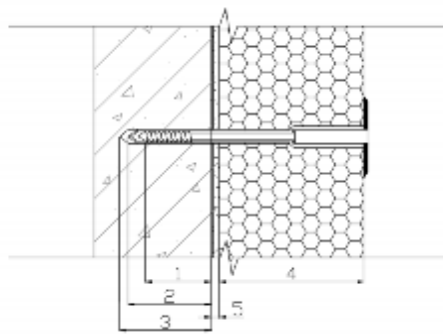
1—有效锚固深度；2—名义锚固深度；3—钻孔深度；4 保温层厚度；5—尺寸偏差
