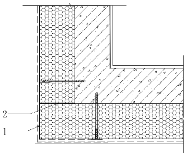
图 B.0.13 阳角处增强做法
