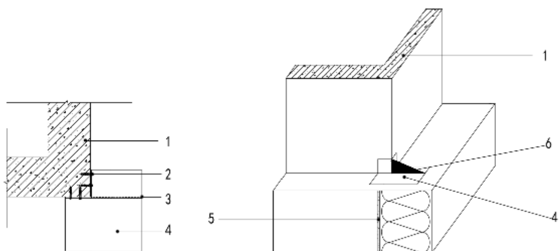
图B.0.7 阳角托架安装
