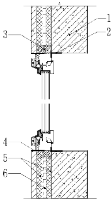
图 B.0.18 装配式建筑外窗安装
