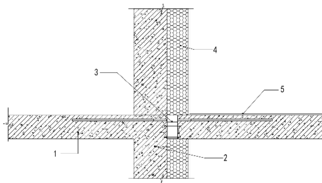
图 B.0.3 阳台板断热桥承重连接件做法
