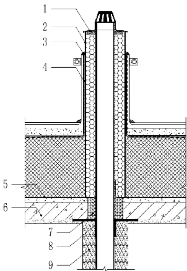
图 B.0.20 出屋面管道做法
