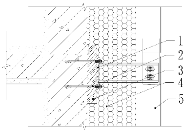
图 B.0.29 幕墙光伏系统断热桥做法
