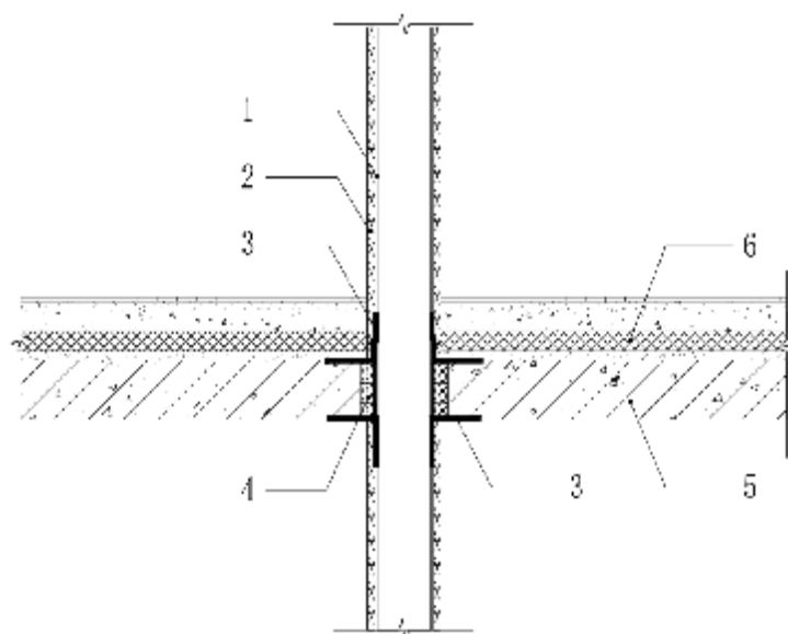
图 B.0.22 穿楼面管道断热桥做法
